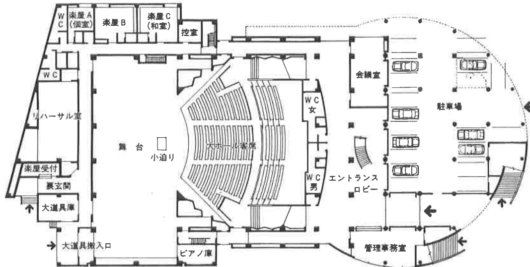
▲ 1階平面図
