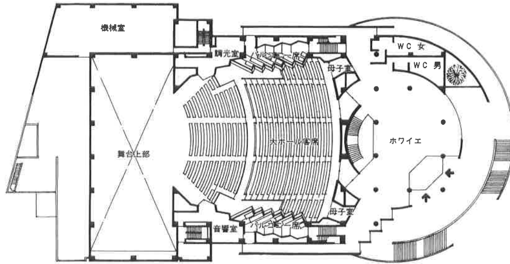
▲ 2階平面図
